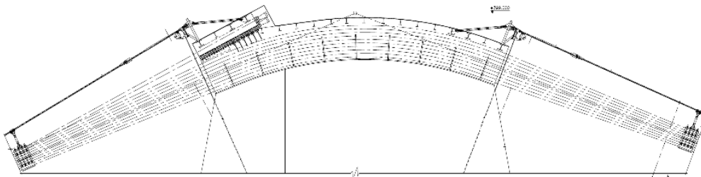
Fig. 18 - Collari per mantenimento forma cavo in prossimità della sella di sommità torre, PD 2011 Ponte di Messina
