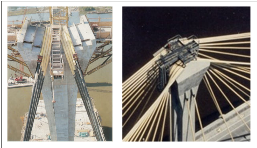
Fig. 20 - Selle di sommità antenna di ponti strallati
