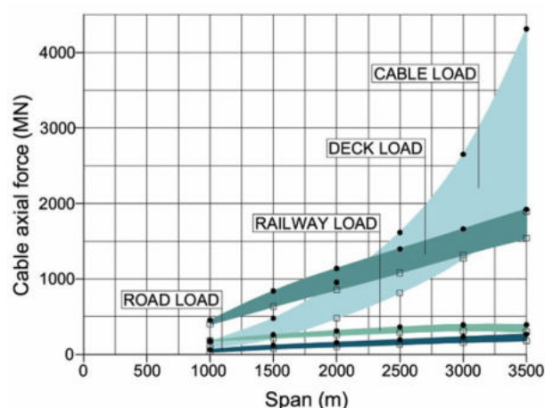
Fig. 1 - Andamento del tiro nel cavo principale dovuto alle diverse componenti dei carichi presenti al variare della luce, tratto da Brancaleoni, Diana, Faccioli, Fiammenghi, Firth, Gimsing, Jamiolkowski, Sluszk, Solari, Valensise, Vullo, The Messina Strait Bridge – A Challenge and a Dream, CRC Press, 2009
