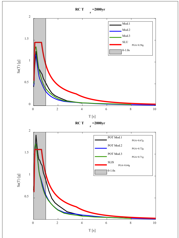
Fig. 28 - (In alto) Spettri a pericolosità uniforme della componente orizzontale calcolati per periodo di ritorno anni lato Calabria (lato Sicilia la situazione è analoga), confrontati con lo spettro di progetto per SLU del progetto definitivo. (In basso) Spettri del picco oltre la soglia calcolato nel sito di Reggio Calabria (RC) per anni e confrontati con lo spettro di progetto per SLIS. Figure tratte dal documento EUROLINK PBW0040.
