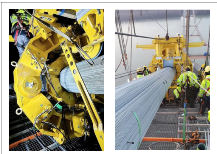
Fig. 16 - Compattazione dei cavi, Ponte sul Danubio a Braila
