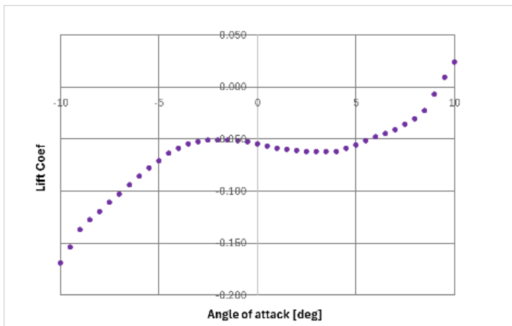
Fig. 4 - Coefficiente di lift, flusso laminare, configurazione di servizio, condizione di traffico 1
