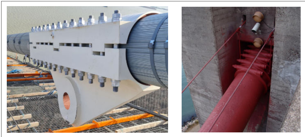
Fig. 17 - A sinistra Collare per collegamento ai pendini, Ponte sul Danubio a Braila; a destra Collare per mantenimento forma cavo, Golden Gate Bridge
