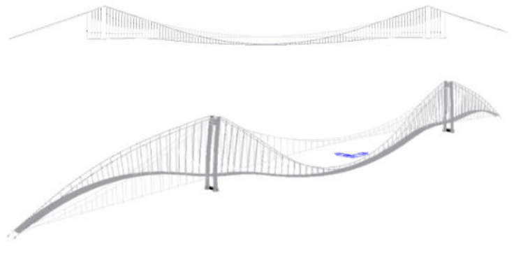
Fig. 2 - Deformate verticali a parità di carico: Ponte sullo Stretto (alto), ponte 1120 m di luce (basso)
