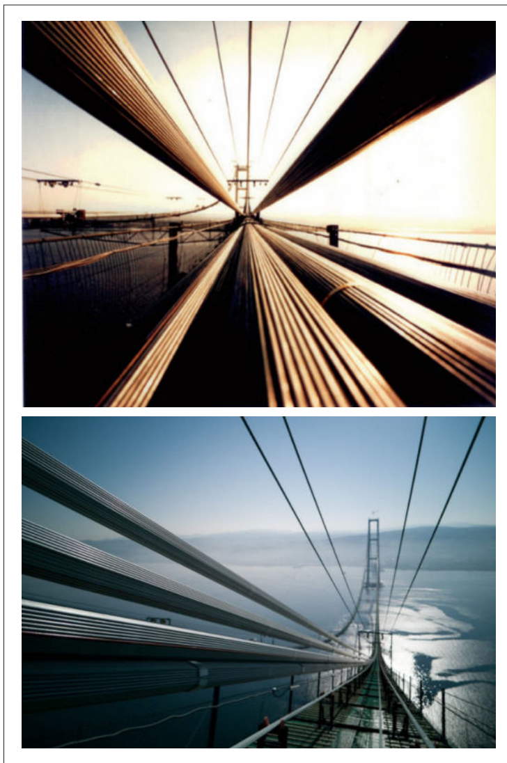
Fig. 15 - In alto funi elementari realizzate con Aerial Spinning, Ponte sull'Humber; in basso, funi elementari realizzate con PPWS, Ponte "1915"
