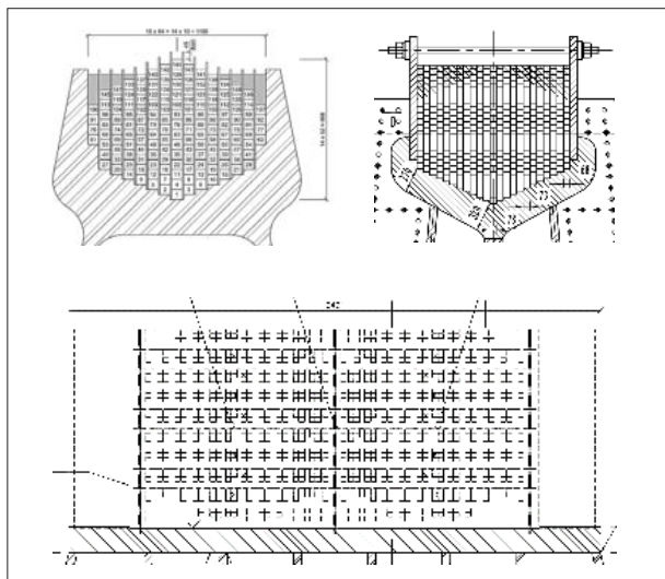
Fig. 23 - Confronto fra differenti concezioni di sella – in alto a sinistra ponte di Canakkale (sella convenzionale); in alto a destra la sella del ponte ShiZiYang, 374 funi, diametro cavo 1486mm; in basso P.D. ponte sullo Stretto di Messina (sella a celle singole)
