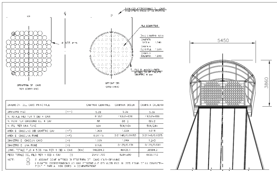
Fig. 21 - Caratteristiche del cavo principale e sezione delle selle - Progetto di Massima 1992
