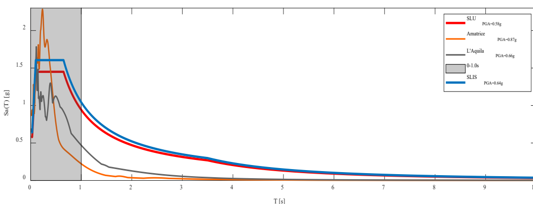
Fig. 27 - Spettri di progetto per SLU e SLIS per il lato Calabria (lato Sicilia la situazione è analoga), e spettri di risposta con la massima PGA registrata durante i terremoti di L'Aquila 2009 e Amatrice 2016
