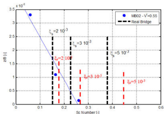
Fig. 6 - Risposta in regime stazionario: oscillazione di ampiezza adimensionalizzata, configurazione MB02, moto flessionale in funzione del Numero di Scruton Number
