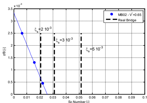
Fig. 8 - Risposta in regime stazionario: oscillazione di ampiezza adimensionalizzata, configurazione MB02, moto torsionale in funzione del Numero di Scruton Number
