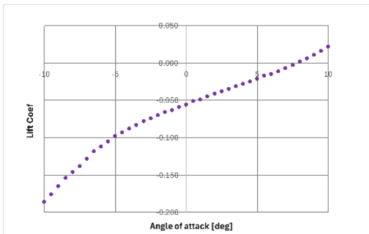
Fig. 5 - Coefficiente di lift, flusso turbolento, configurazione di servizio, condizione di traffico 1
