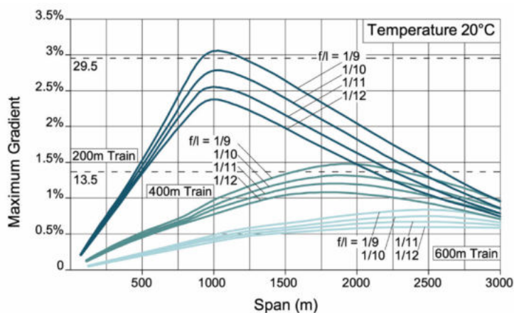
Fig. 3 - Variazione della massima pendenza longitudinale in funzione della luce, tratto da Brancaleoni, Diana, Faccioli, Fiammenghi, Firth, Gimsing, Jamiolkowski, Sluszka, Solari, Valensise, Vullo, The Messina Strait Bridge – A Challenge and a Dream , Volume, CRC Press, 2009
